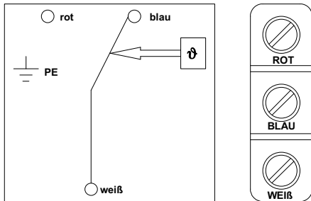
Anschlußschaltbild
