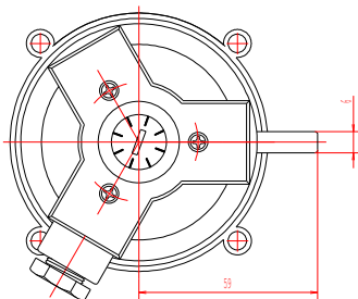
Differenzdruckwächter
