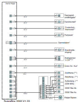
Abbildung 1: Verdrahtungsplan
